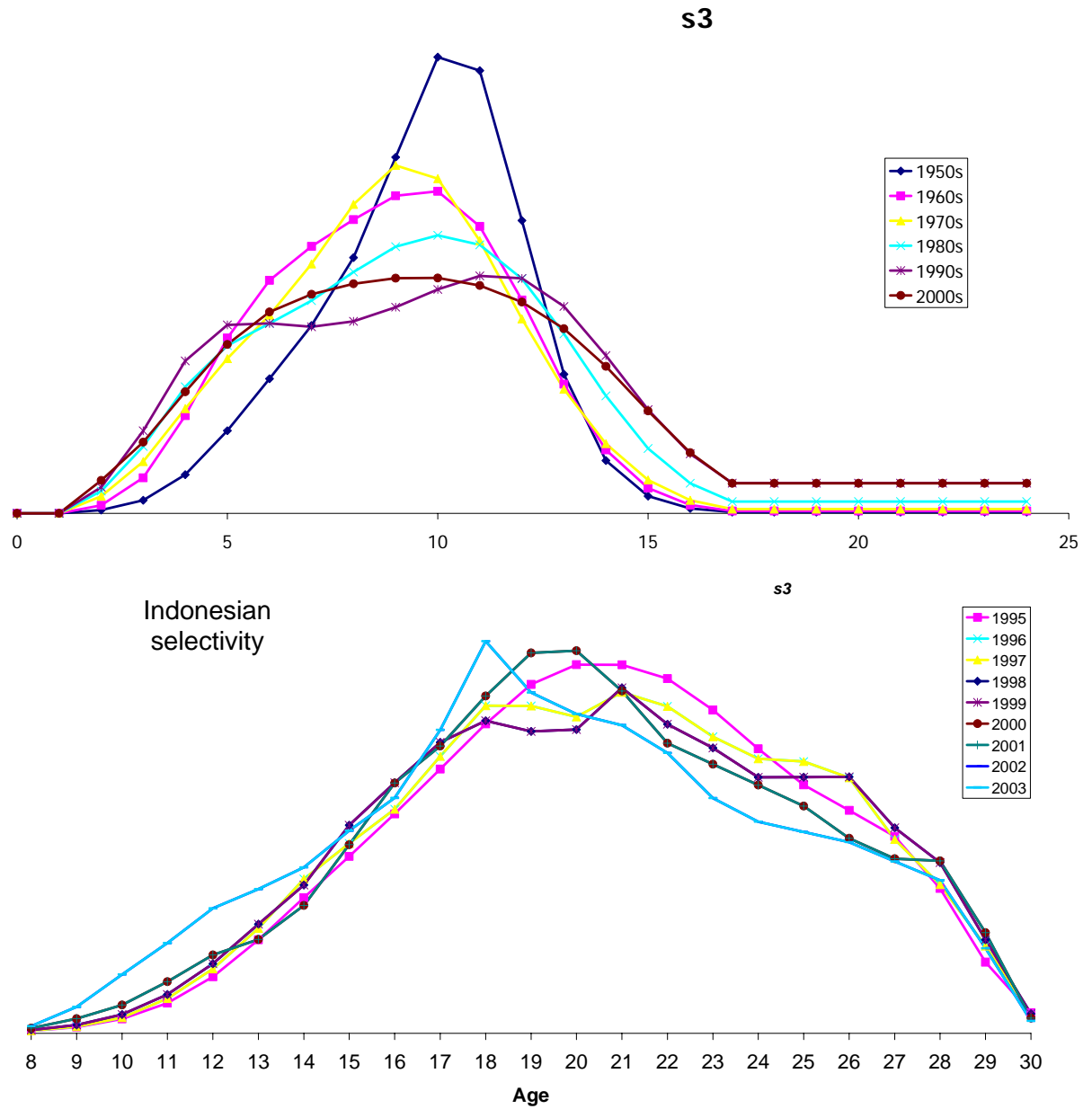
図3 はえ縄1漁業(上のパネル)とモデルs3の下でのインドネシアの漁業(下のパネル)の選択性
